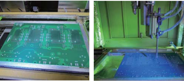
PCBA喷涂前蓝光检测
